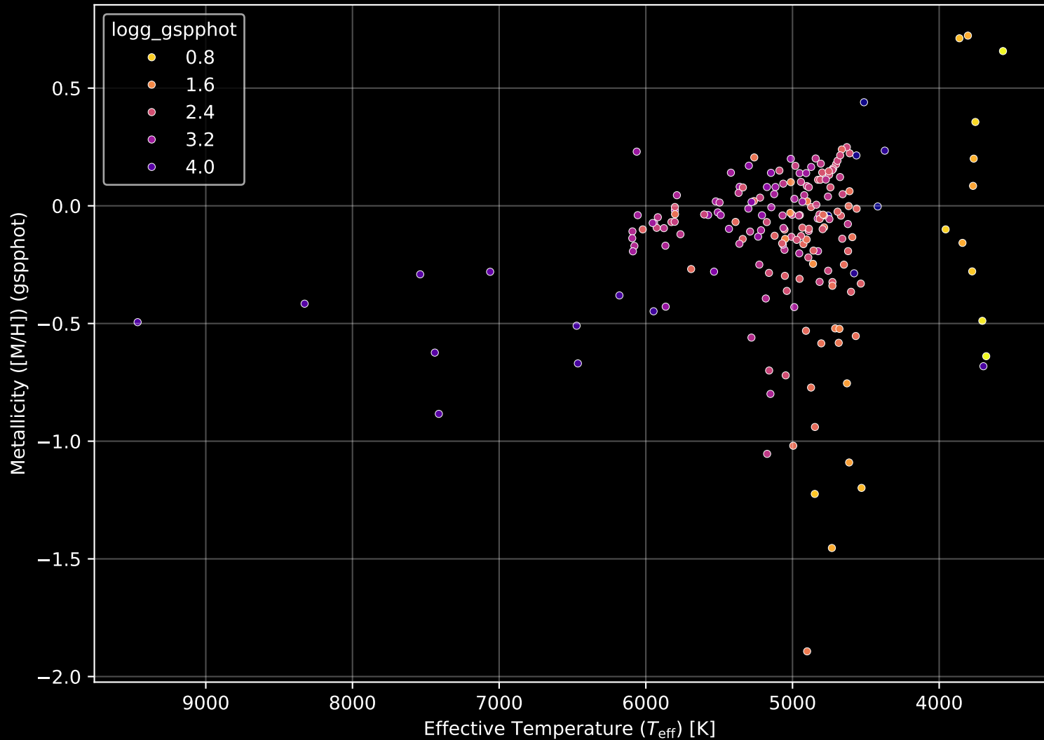
APOGEE DR17 Field: [020+14] Stellar Population Parameters (n= 195)
